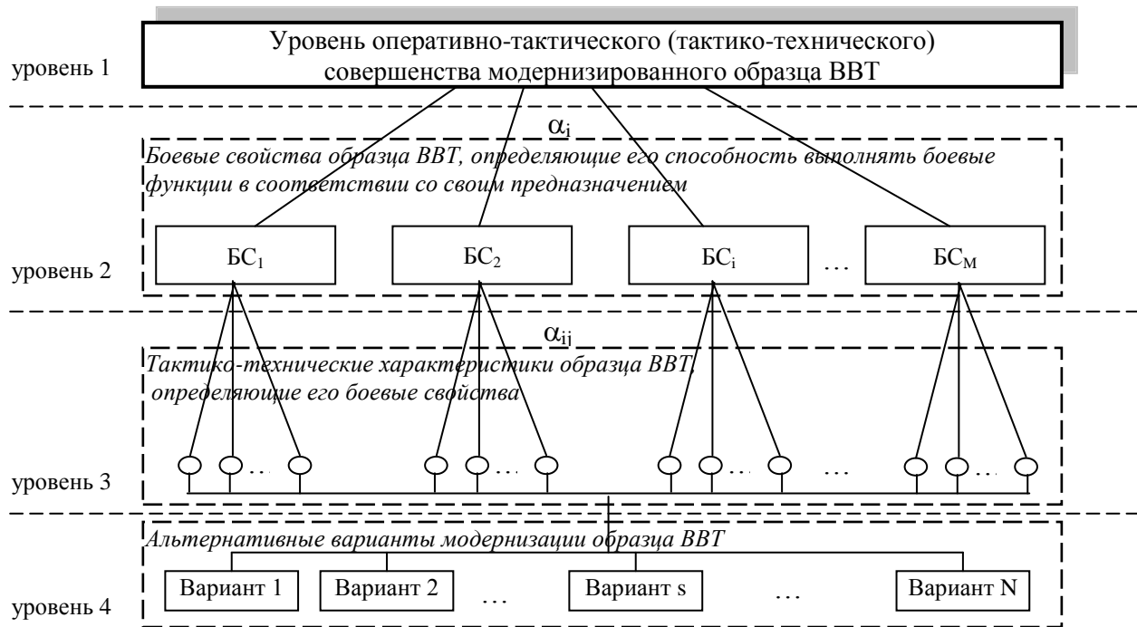
Рис. 1. Декомпозиція задачі оцінювання рівня технічного досконалості модернізованого зразка ВВТ
