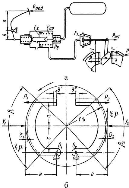
Рис. 2. Схема пневматичного приводу РГС: а – загальної конструкції; б – сил, що діють на колодки гальмівного механізму
