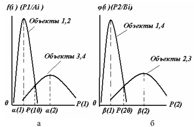
Рис. 2. Плотности вероятностей признаков: а – распознавания объектов 1, 2 и 3 4 классов; б – распознавания признаков объектов 1, 4 и 2, 3о классов
