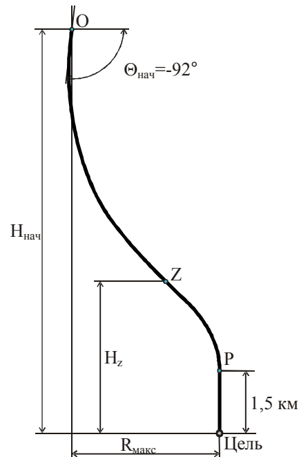
Рис. 1. Схема маневрирования
