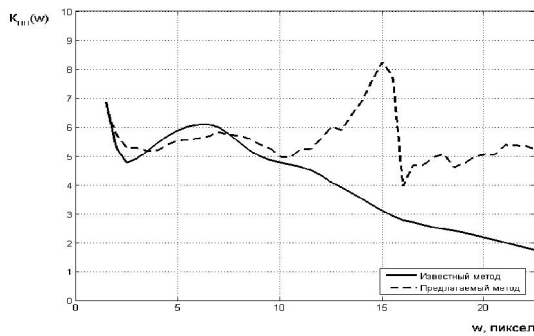
Рис. 5. Зависимость коэффициента подавления помехи K_{п}(w) от полуширины окна обработки
