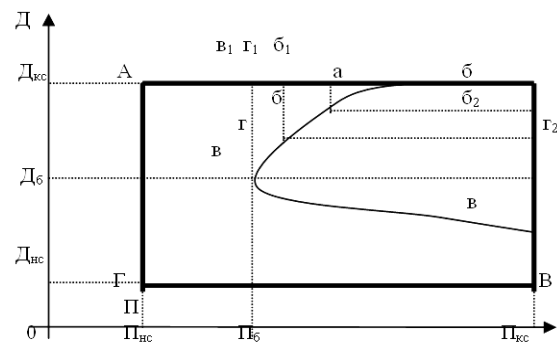
Рис. 2. Проєкції b_1, v_1, g_1 точок берегової лінії розташовуються поза основою берега, рівнобіжною осі пеленга
