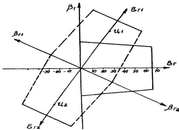
Рис. 1. Принцип обнуление азимута путем разворота антенны по крену
