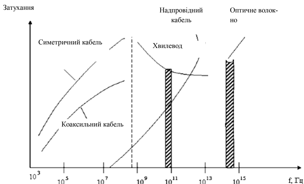
Рис. 1. Частотна залежність згасання різних ліній передачі
