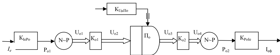
Рис. 2. Приклад параметричної структурної схеми
