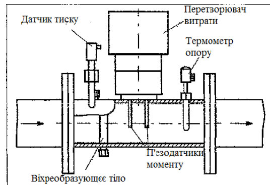
Рис. 2. Первинний перетворювач витрати "ІРГА-РВ"
