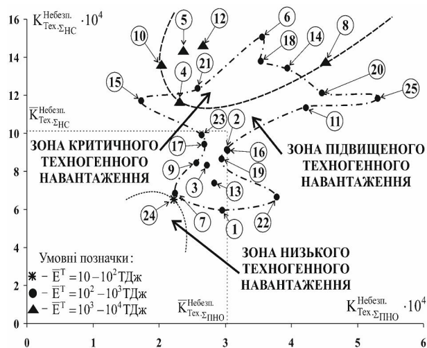
Рис. 8. Графічні залежності між показником техногенної небезпеки за сумарною кількістю потенційно небезпечних об'єктів на душу населення ( K_{\text{Тех.}\Sigma\text{ПНО}}^{\text{Небезп.}} ) та показником техногенної небезпеки за сумарною кількістю надзвичайних ситуацій на душу населення ( K_{\text{Тех.}\Sigma\text{НС}}^{\text{Небезп.}} ) в умовах споживання регіонами України (нумерація областей наведена в алфавітному порядку і відповідає рис. 3) середньодобової енергії техногенного походження ( \bar{E}^T )
