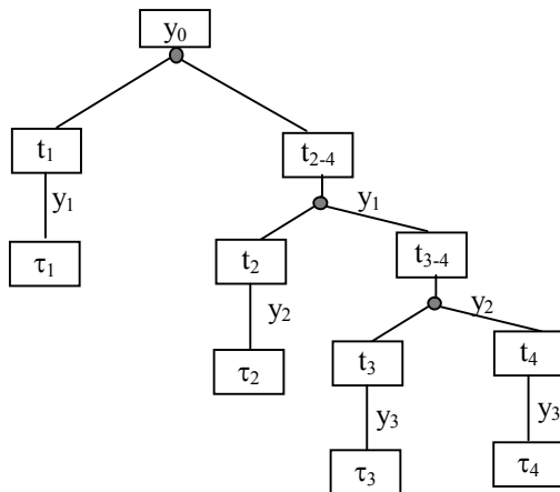
Рис. 2. Структурна схема усунення несправностей після об'єднання елементарних операцій:
