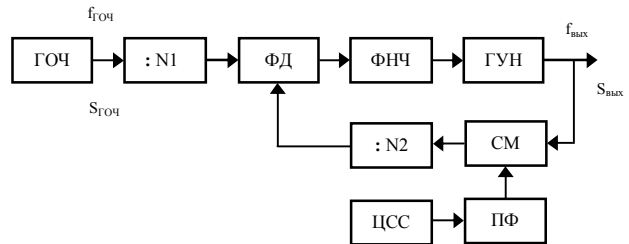
Рис. 4. Комбинированный синтезатор со смещением частоты ГУН
