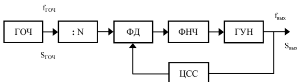
Рис. 2. Комбинированный синтезатор с использованием ЦСС как делителя частоты в системе ФАПЧ
