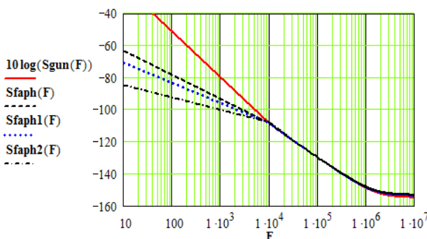
Рис. 6. Зависимость ОСП шумов ФАПЧ от частоты отстройки при различных коэффициентах деления N2:
