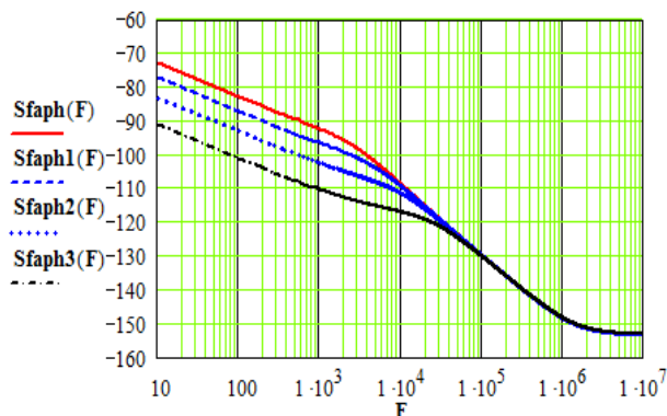
Рис. 7. Зависимость ОСП шумов ФАПЧ от частоты отстройки при различных коэффициентах умножения системы ФАПЧ ( N_2/N_1 ): N_2/N_{1_{faph}} = 5 ; N_2/N_{1_{faph1}} = 4 ; N_2/N_{1_{faph2}} = 2 ; N_2/N_{1_{faph3}} = 1
