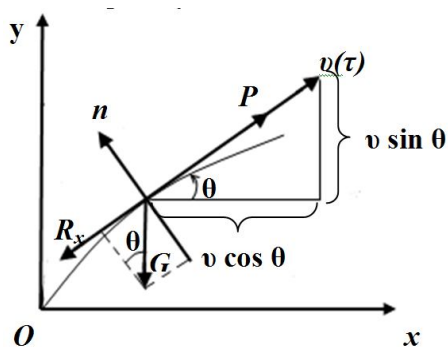
Рис. 1. Сили, що діють на ракету
