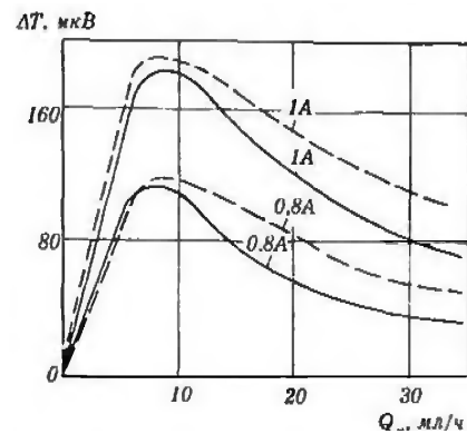
Рис. 2. Різниця температур \Delta T (в мкВ ТЕРС) в залежності від витрати води (витрата 10 мл/год відповідає швидкості 0,346 мм/с), сили струму в нагрівачі та місць розташування термоперетворювачів: — для наближеної термобатарей; - - - для віддаленої термобатарей
