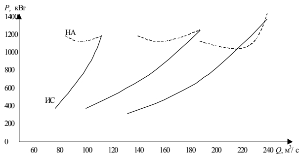
Рис. 1. Графіки потужності при регулюванні відцентрового вентилятора ВЦЦ-32 направляющим апаратом (НА) і змінною швидкості (ІС)
