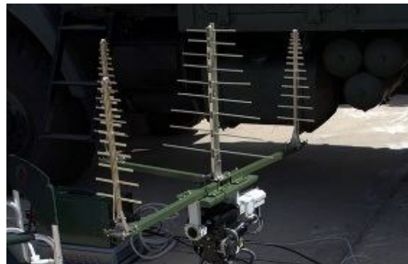
Рис. 4. Антенна станции РЕБ «Красуха-4»
