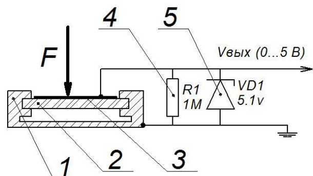
Рис. 1. Измерительная схема
