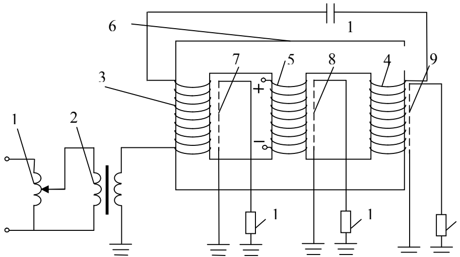
Рис. 1. Схема резонансного пристрою контролю часткових розрядів
