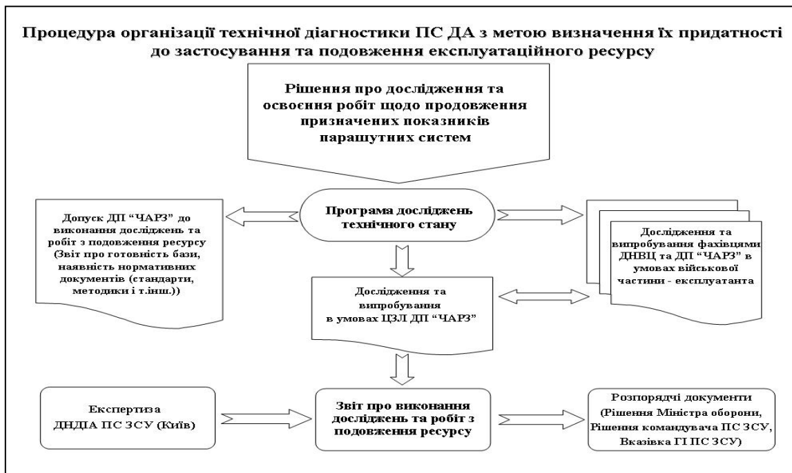
Рис. 2. Процедура організації ТД ПС ДА з метою визначення їх придатності до застосування та подовження експлуатаційного ресурсу
