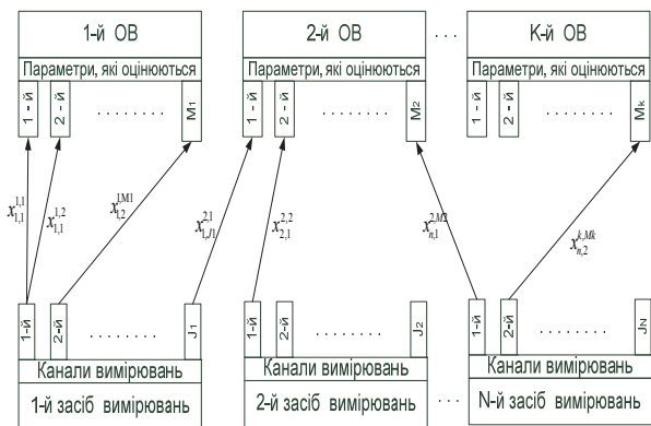
Рис. 1. Схема варіанту застосування засобів ПВОК для оцінки параметрів об'єктів випробувань
