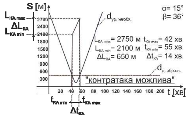
Рис. 9. Результати розрахунку L_{КА} і t_{КА} , при \alpha = 15^\circ , \beta = 36^\circ
