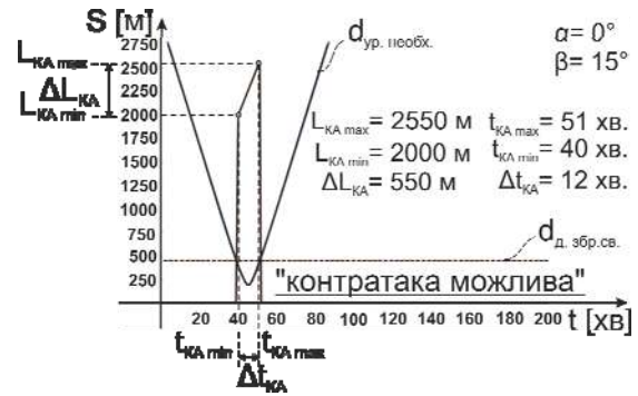
Рис. 7. Результати розрахунку L_{КА} і t_{КА} , при \alpha = 0^\circ , \beta = 15^\circ
