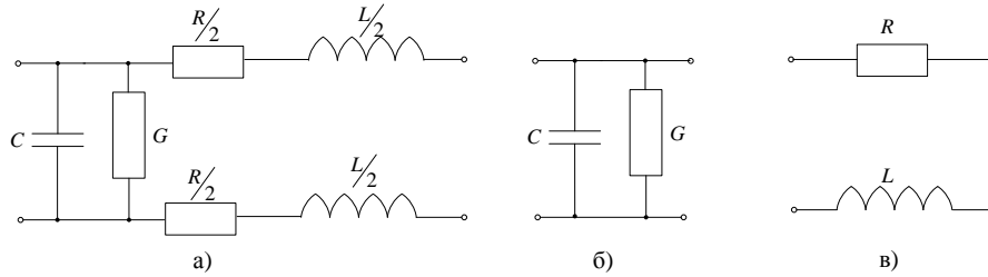
Рис. 3. Повна (а) та спрощені схеми заміщення знеструмленої «чистої» абонентської телефонної лінії в режимі холостого ходу (б) і короткого замикання (в) на віддаленому кінці
