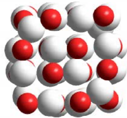
Рис. 3. Структура невеликого (32 молекули, 1,01 нм) кристалу MgO змодельована напівемпіричним методом РМЗ.
