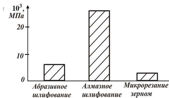
Рис. 4. Значения энергоемкости обработки \sigma для разных условий обработки
