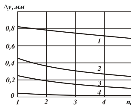
Рис. 2. Зависимость \Delta y от n_0 :
