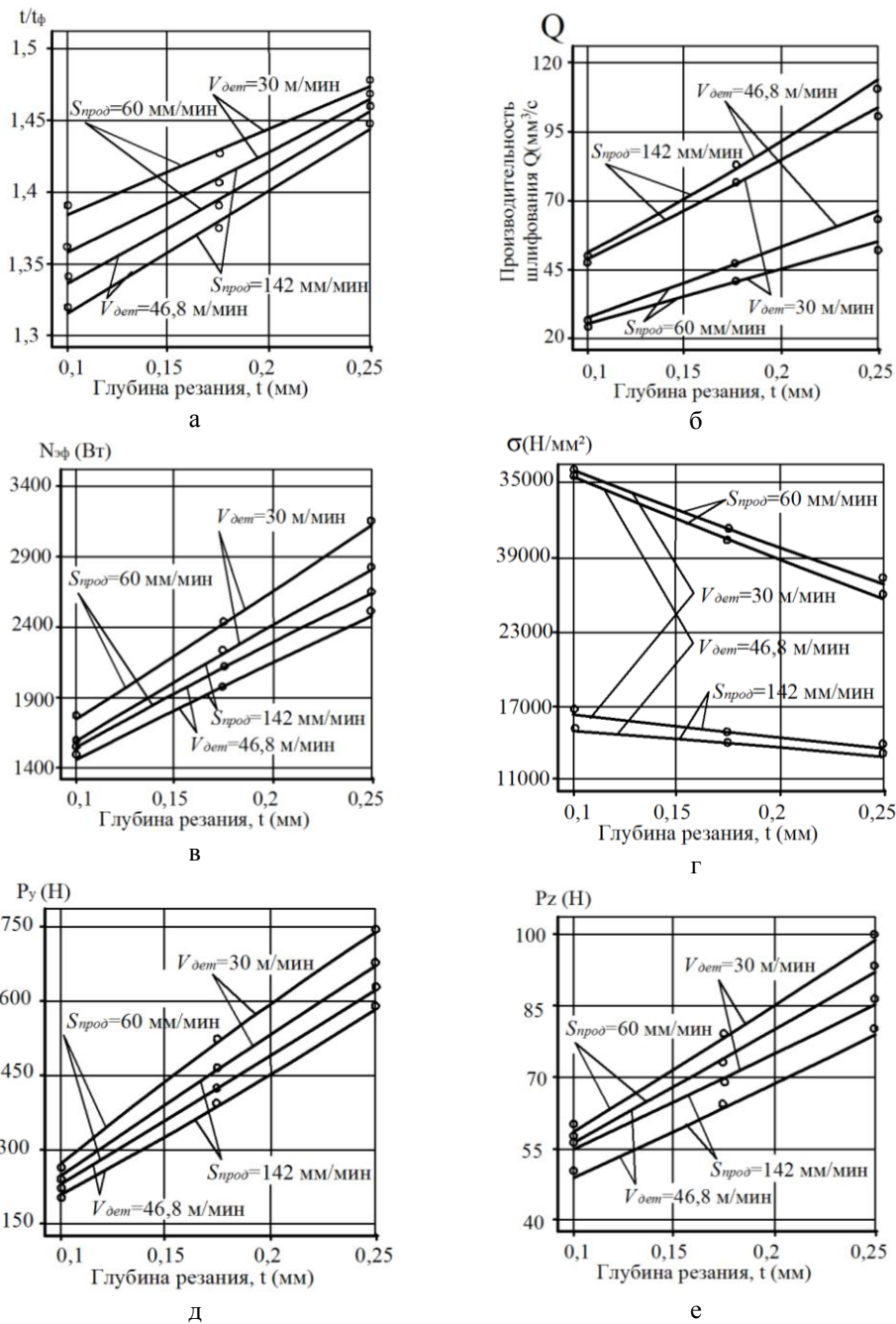
Рис. 3. Зависимости t/t_{ф} (а), Q (б), N_{эф} (в), \sigma (г), P_y (д) и P_z (е) от глубины шлифования t
