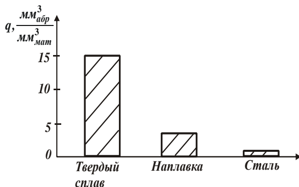
Рис. 5. Значения удельного износа круга q при шлифовании разных материалов
