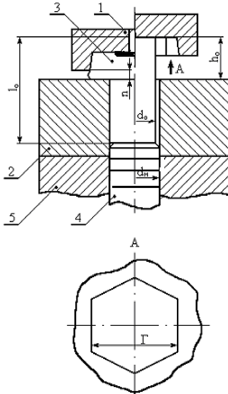
Рисунок 2 – Загальний вид експериментального штамп: 1 – пуансон; 2 – матриця; 3 – корпус; 4 - виштовхувач.
