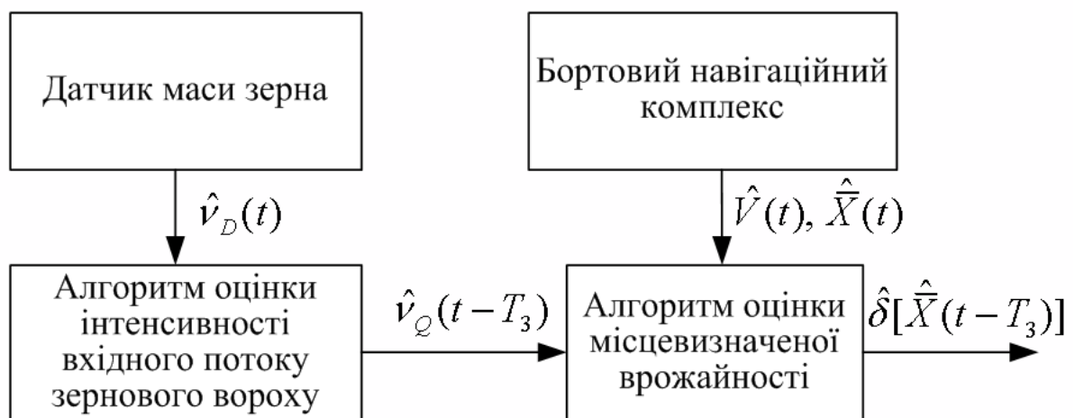
Рисунок 6 - Структурна схема типової бортової системи картографування врожайності
