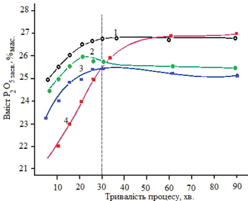
Рисунок 3 – Залежність вмісту P_2O_{5\text{засв.}} від тривалості процесу при різних концентраціях HNO_3 при температурі t = 75^\circ\text{C}
