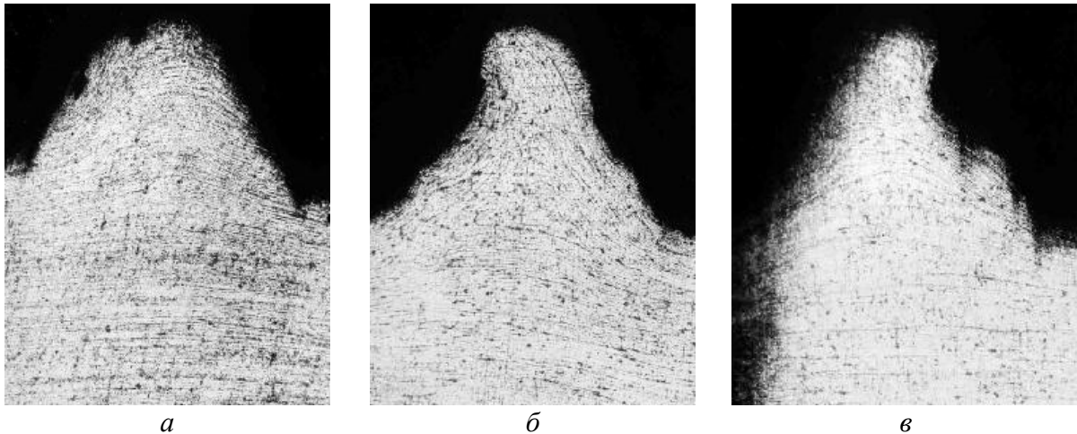
Рисунок 2 – Макроструктура зубьев резьбы: а – зуб резьбового профиля гайки высотой 8 мм; б – зуб резьбового профиля гайки высотой 4,5 мм; в – зуб резьбового профиля гайки высотой 4 мм
