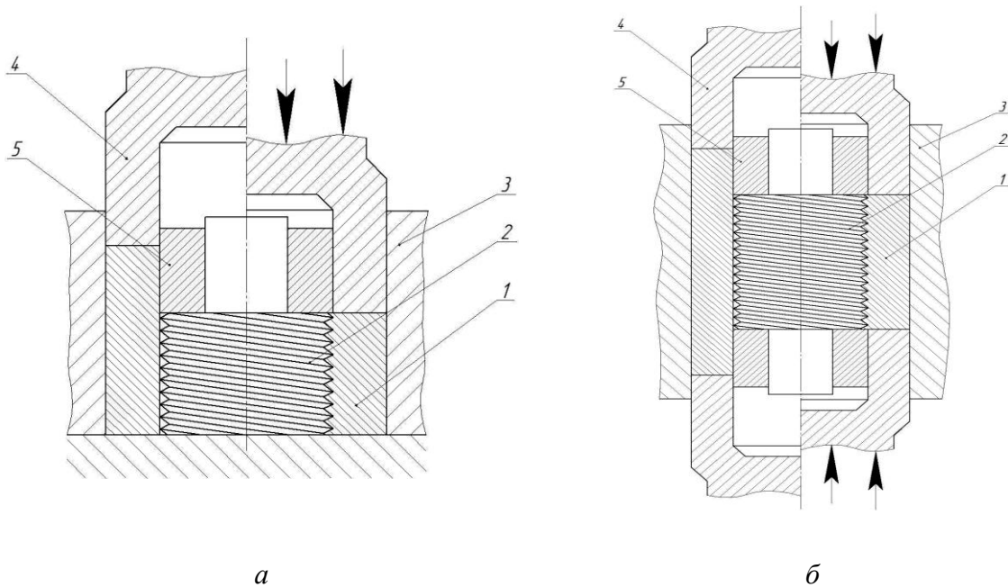
Рисунок 1 – Способ бокового выдавливания резьбы (1 – заготовка; 2 – резьбовая оправка; 3 – матрица; 4 – пуансон; 5 – направляющая втулка): а – односторонняя схема выдавливания; б – двусторонняя схема выдавливания
