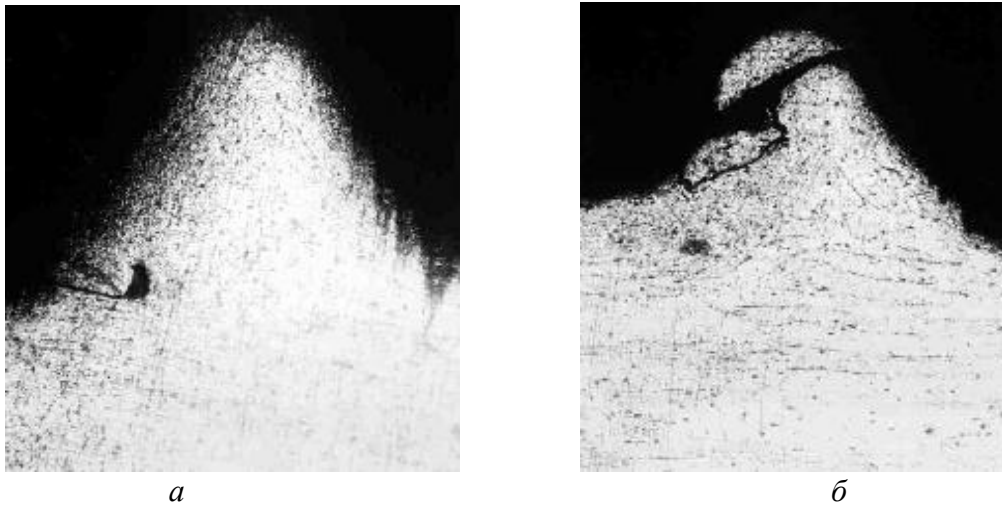
Рисунок 5 – Дефекты резьбового профиля: а – микротрещина у основания зуба резьбового профиля; б – скол вершины зуба резьбового профиля
