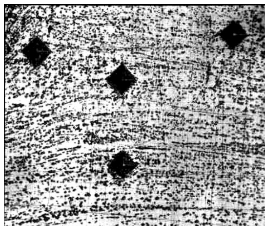
Рисунок 3 – Отпечатки алмазной пирамиды
