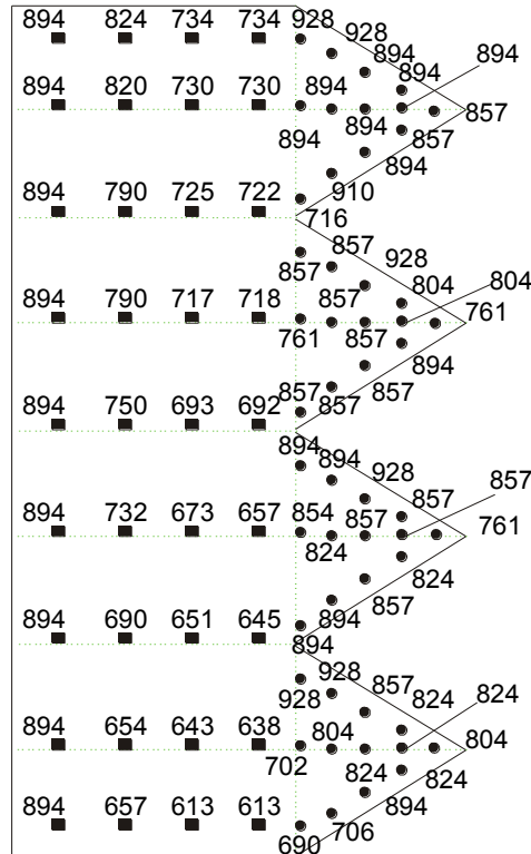
Рисунок 4 – Микротвердость ( H_{10} ) профиля резьбы, полученной боковым выдавливанием, высота гайки 4 мм
