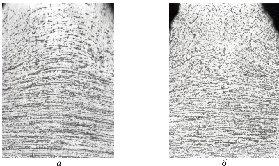
Рисунок 6 – Макроструктура профиля стенки и части резьбы гайки
