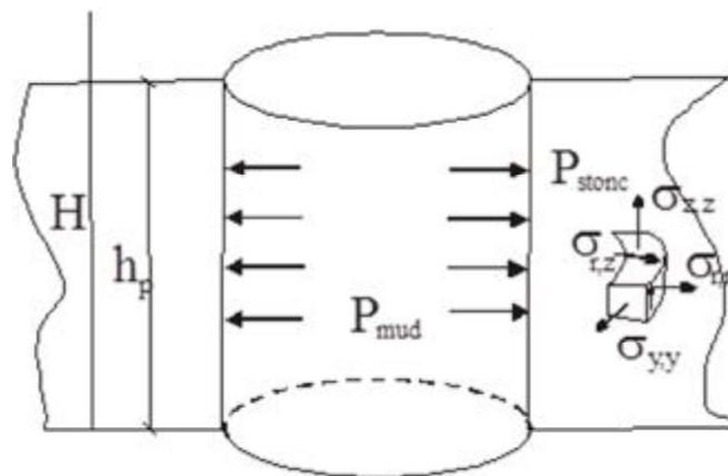
Рис. 2. Розрахункова схема задачі С.Г. Лехницького
