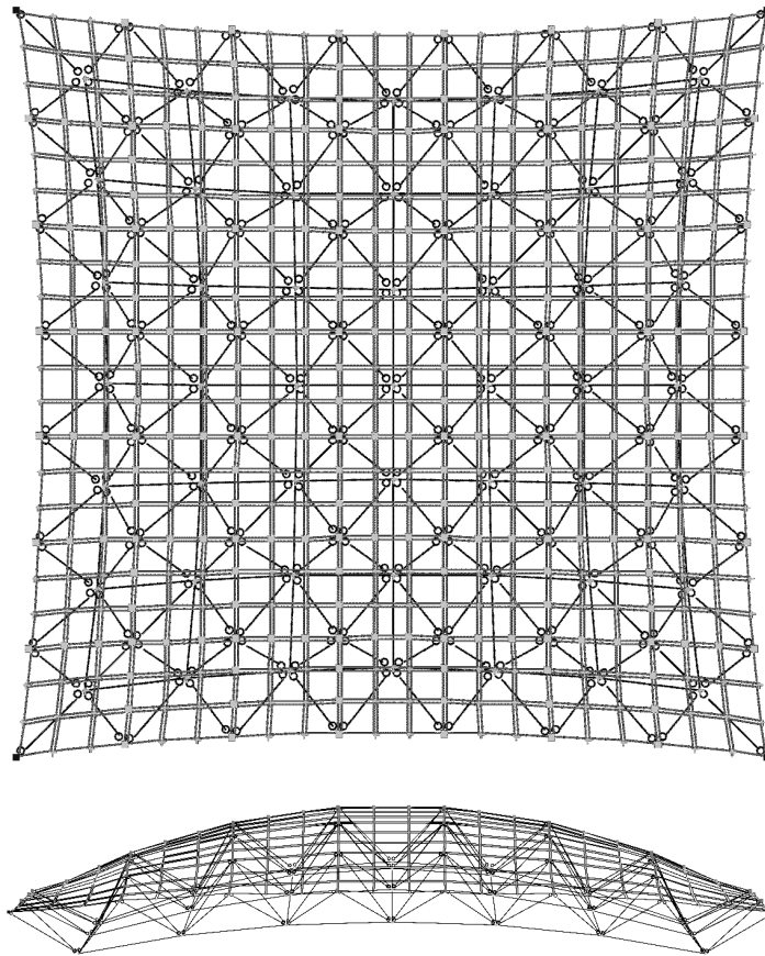
Рис. 5. Деформована схема оболонки
