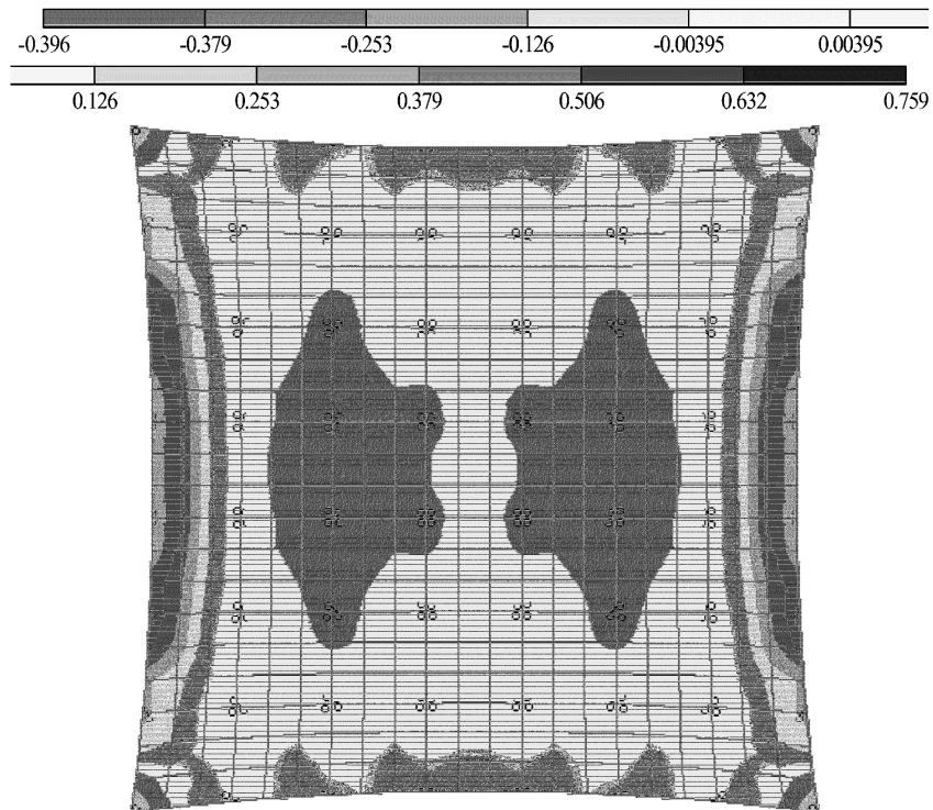
Рис. 6. Ізополя напружень N_u , МПа
