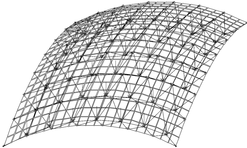
Рис. 3. Схема завантаження оболонки у вузлах нижнього пояса
