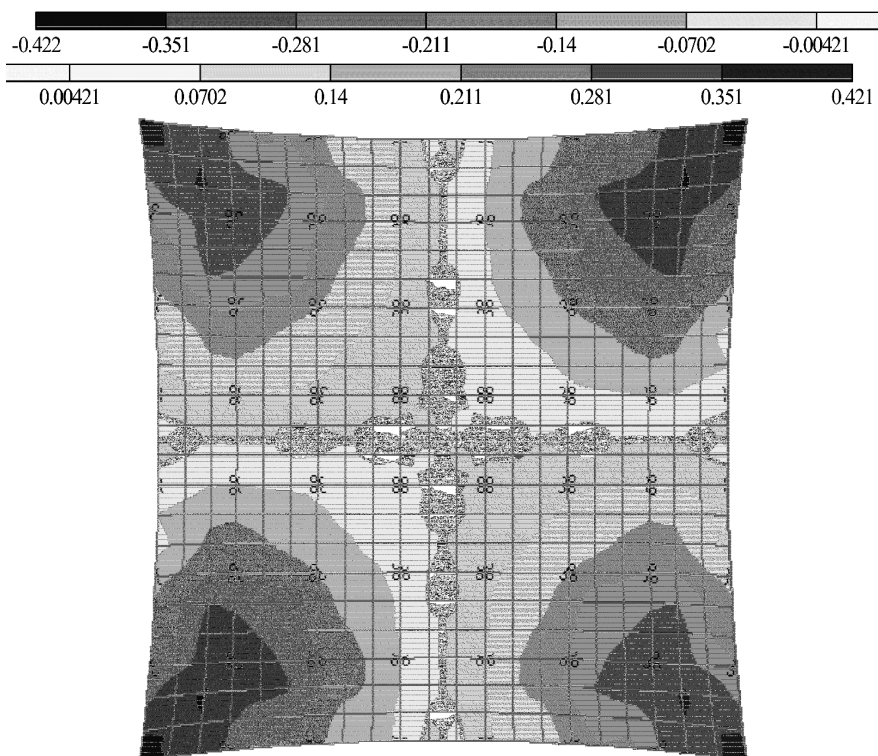
Рис. 7. Ізополя напружень T_{xy} , МПа
