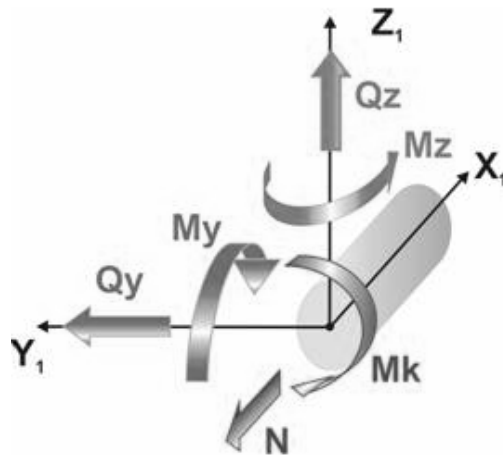
Рис . 1. Зусилля в перерізі стрижня
