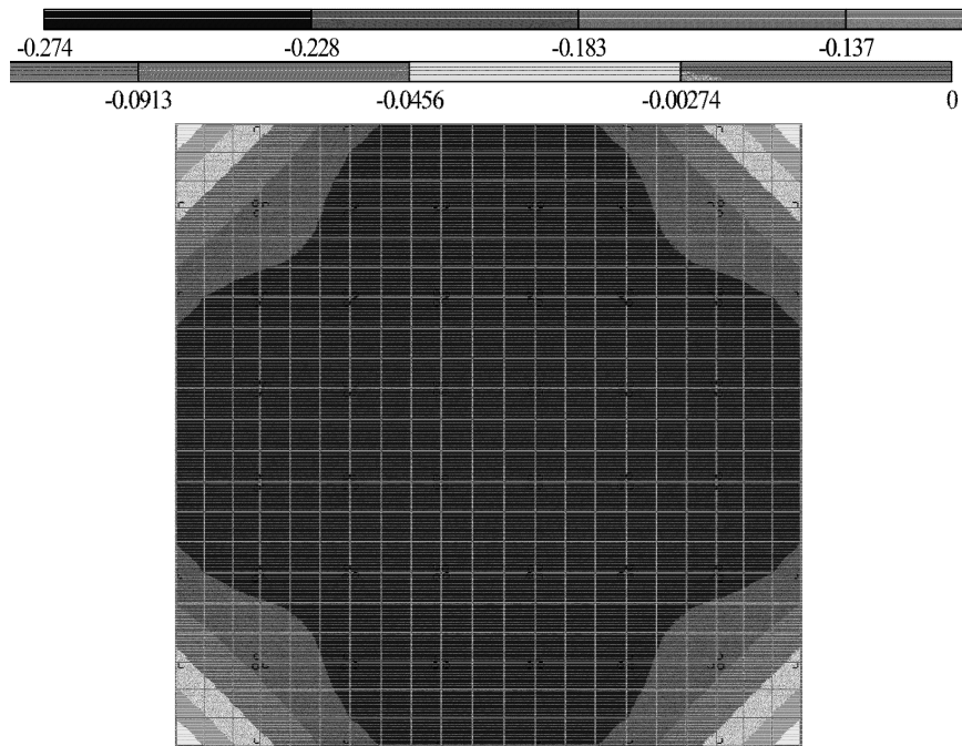
Рис. 8. Вертикальні переміщення Z , мм
