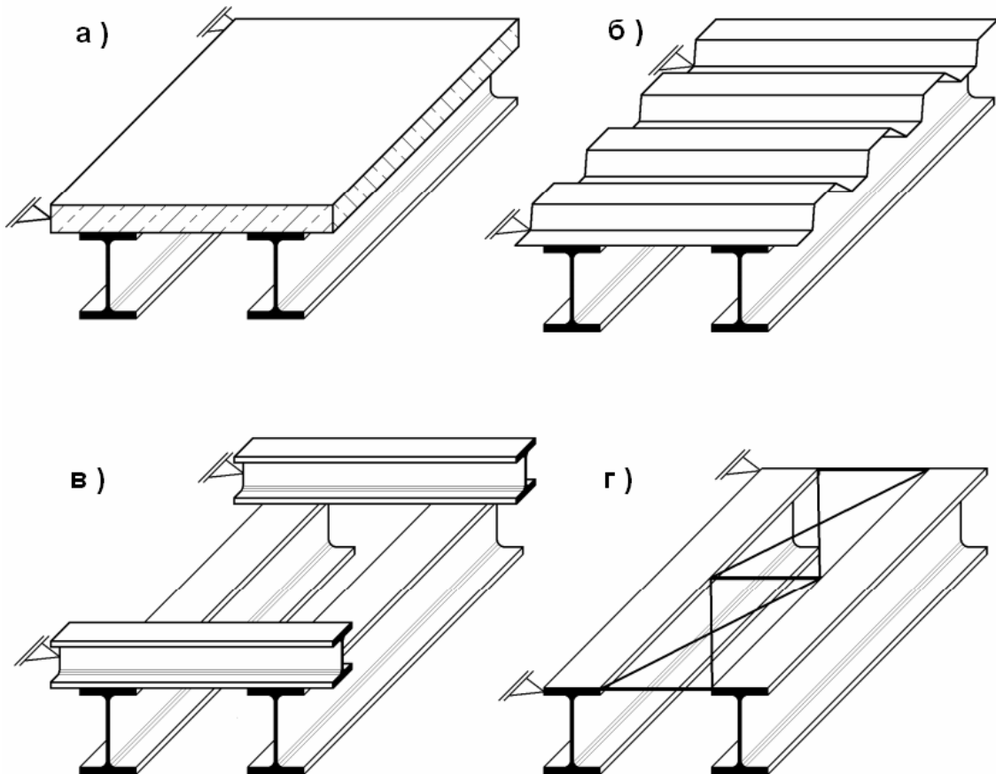
Рис. 1. Різновиди розкріплення сталевих балок за допомогою стабілізуючих конструкцій: а) залізобетонної плити; б) сталевого профільованого настилу; в) прогонів; г) хрестових в'язей
