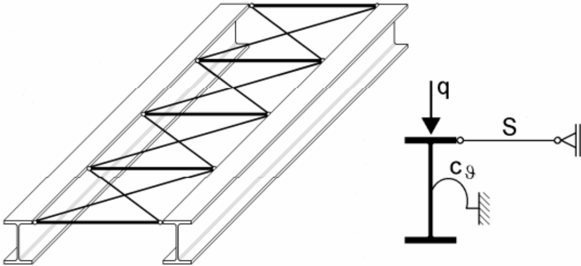
Рис. 2. Схема розташування дискретних в'язей по довжині сталевих балок і умовний вигляд поперечного перерізу сталевих балок із позначенням зсувної (S) і крутильної (с) жорсткостей дискретних в'язей
