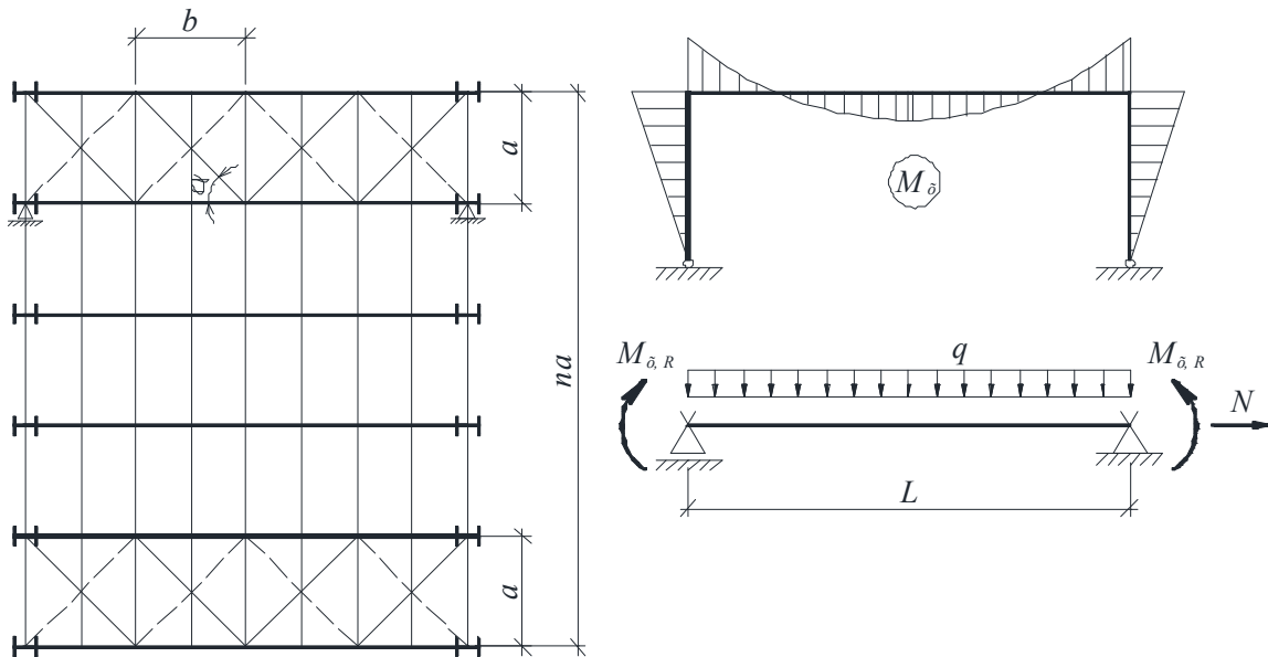
Рис. 3. Розрахункова схема розкріпленої в'язями балки, що слугує ригелем двохпідпорожкової поперечної рами
