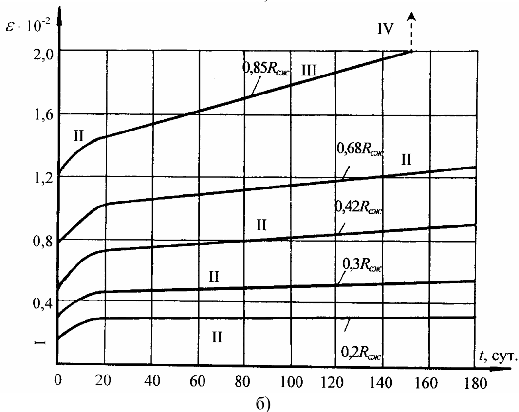
Рис. 3. Диаграммы ползучести акрилового клея при растяжении (а) и сжатии (б)
