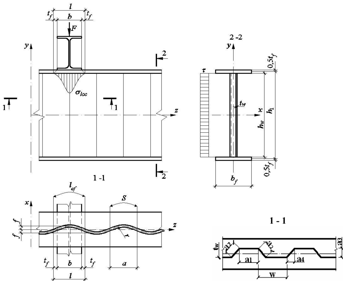
Рис. 1. Схема елемента з хвилястою і трапецієподібною поперечно-гофрованою стінкою
