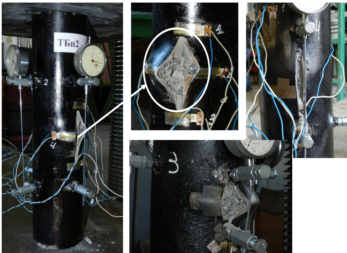
Рис. 1. Характер руйнування дослідних зразків серії ТБп2
