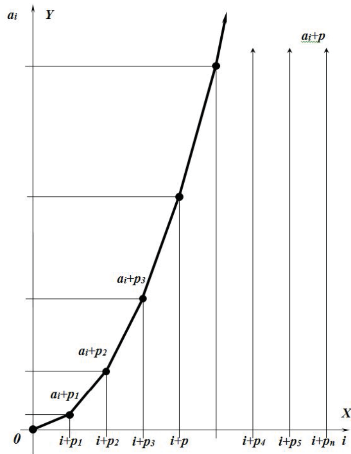
Рис. 1 – Графік числової послідовності a_i = c^i
