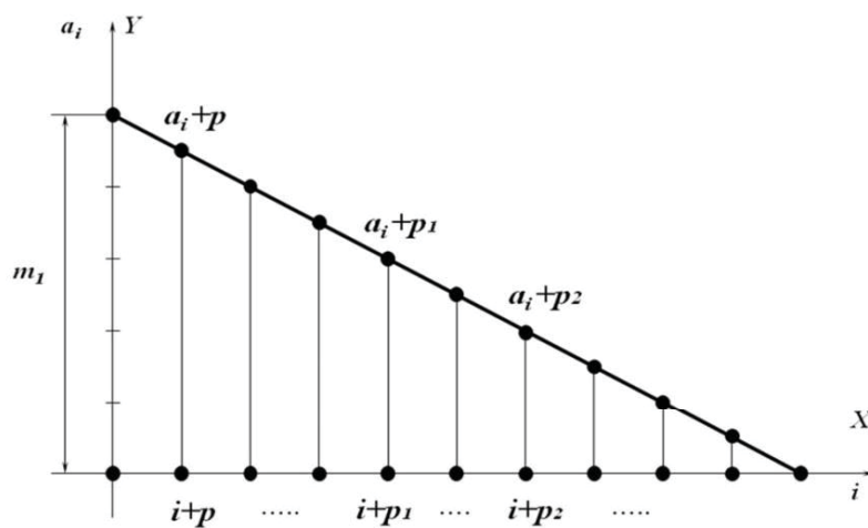
Рис. 4 – Графік числової послідовності a_i = m_0 + m_1 i
