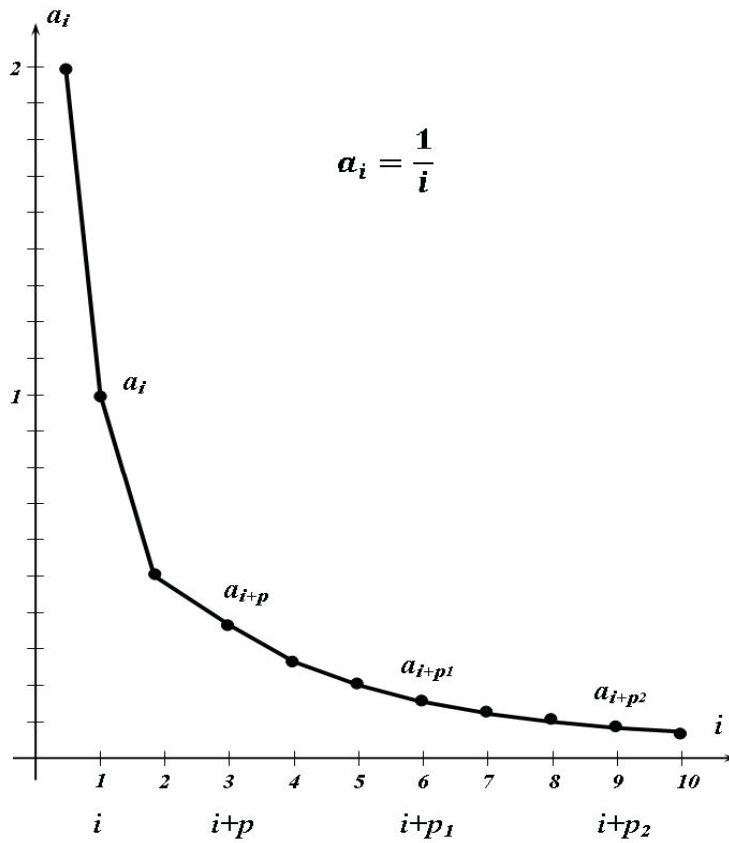
Рис. 3 – Графік дробово-лінійної функції a_i = \frac{1}{i}
