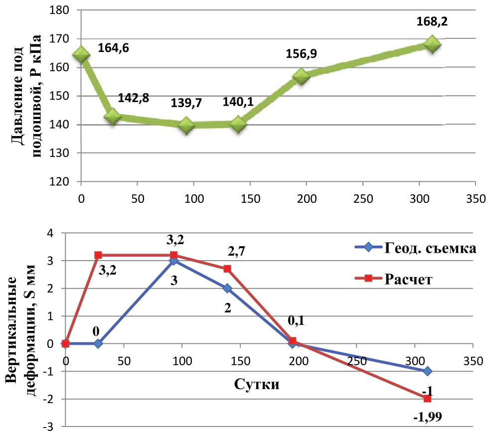
Рис. 7 – График вертикальных деформаций марки М-1
