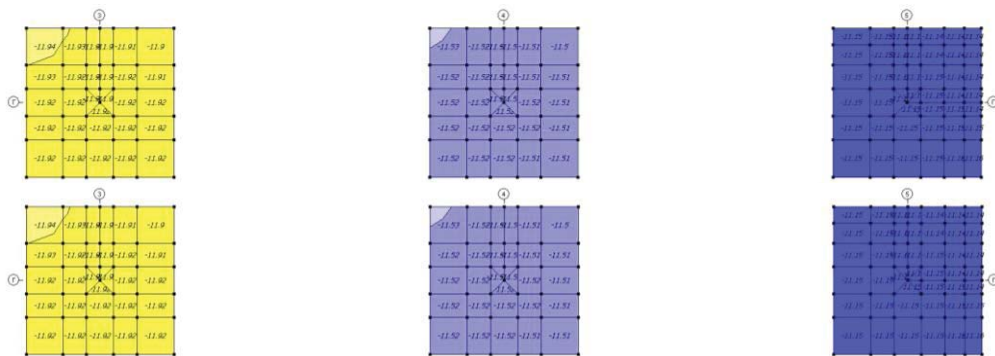
Рис. 8 – Давление под подошвой отдельно стоящих фундаментов, кПа
