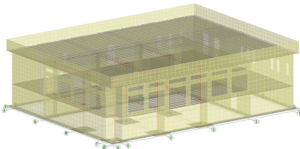
Рис. 3 – Расчетная схема МКЭ здания магазина до реконструкции
