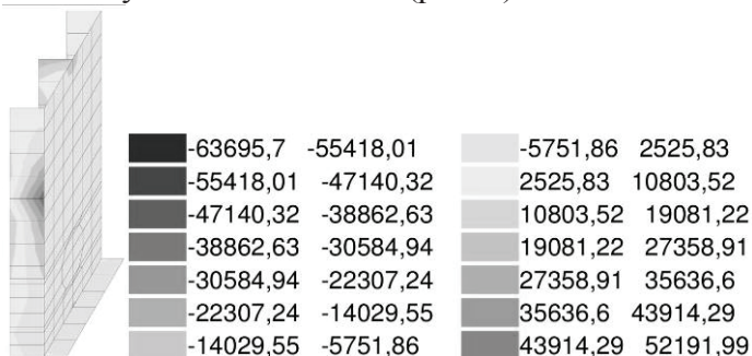
Рисунок 4 – Розподіл напружень N_x ( kH/m^2 ) в опорній частині
