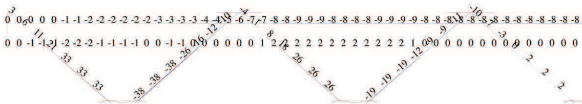
Рисунок 5 – Напруження N ( kH ) в стрижнях
