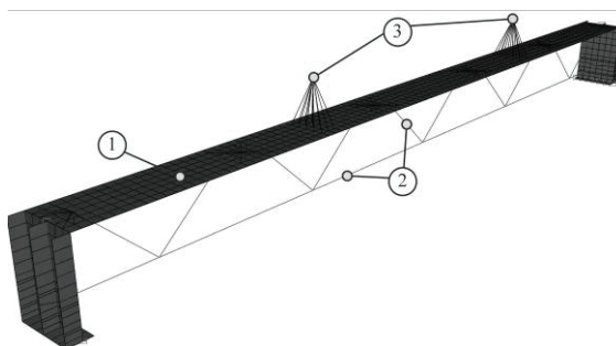
Рисунок 7 – Другий випадок розрахункової скінченноелементної моделі балки: 1 – 3- та 4-кутові СЕ оболонки; 2 – універсальний стрижень; 3 – абсолютно тверді тіла АТТ
