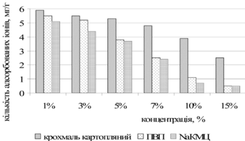
Рис. 1. Залежність адсорбційної здатності таблеток целюліту від виду та концентрації зволожувача
