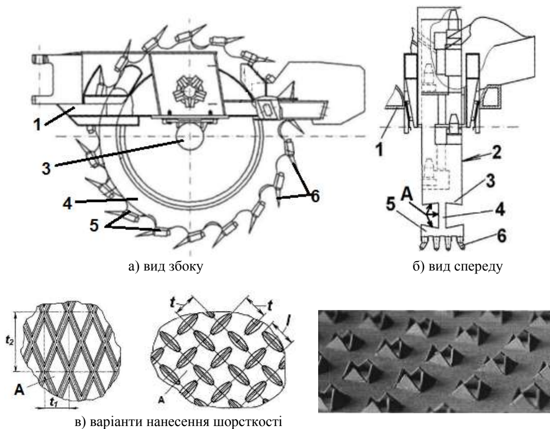
Рис. 2. Конструкція бесківшового роторного робочого органа та варіанти нанесення шорсткості на робочі поверхні ротора:
