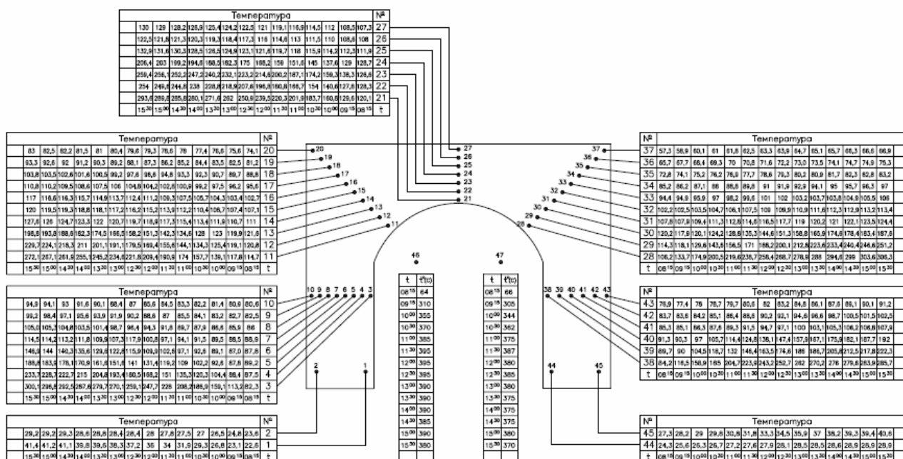
Рис. 3. Схема расстановки термопар в железобетонном фрагменте фундамента №1 с футеровкой бора
