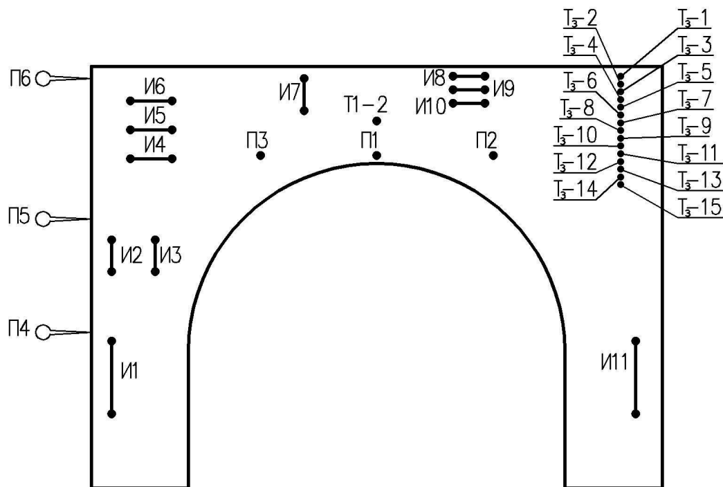
Рис. 4. Схема расстановки индикаторных тензодатчиков И1-И11 на бетон, рычажных тензодатчиков Т1-Т2 на верхней и нижней арматуре, тензодатчиков Тз_1- Тз_15 на бетон и прогибомеров П1-П6 в фрагменте фундамента №1
