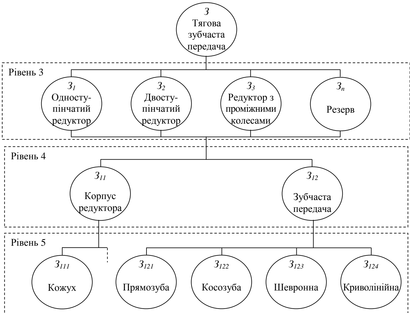
Рис. 2. Декомпозиційний склад модуля зубчастої передачі
