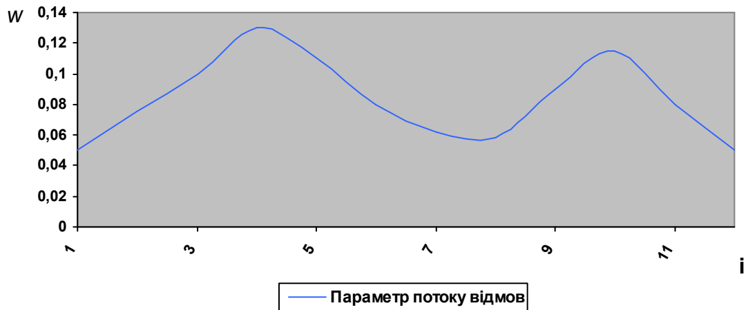
Рис. 1. Графік функції параметру потоку відмов автомобіля УАЗ-3151
