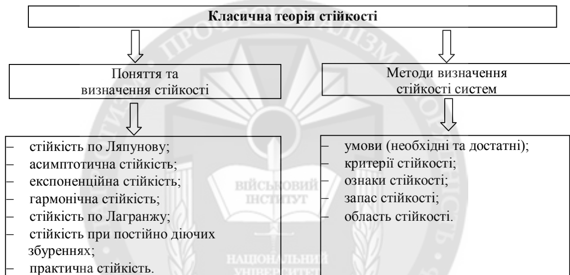
Рис. 1. Класифікація понять класичної теорії стійкості
