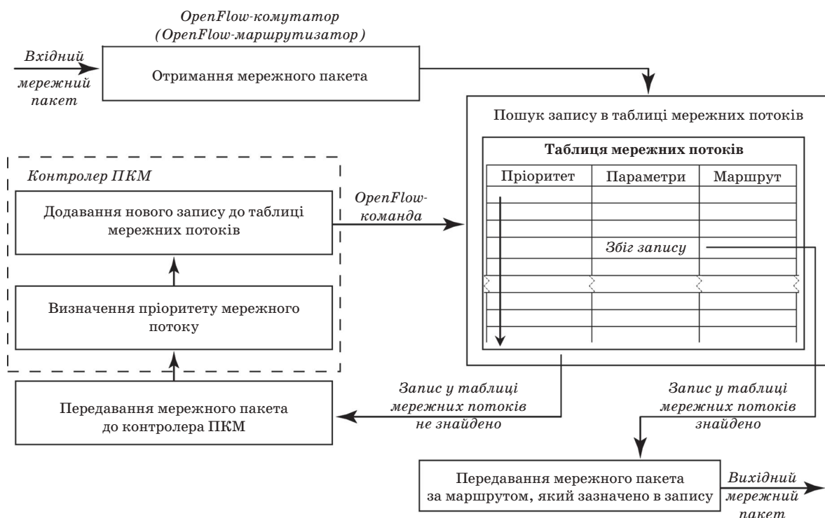
Схема адаптивного управління мережними потоками в ПКМ
