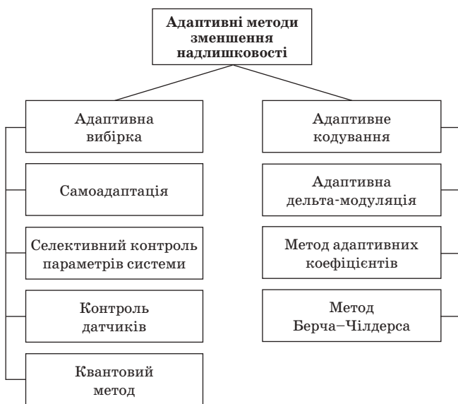
Класифікація адаптивних методів зменшення надлишковості
