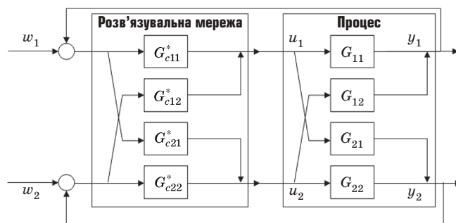
Рис. 2. Розв'язувальна система управління Боксенбома і Гуда
