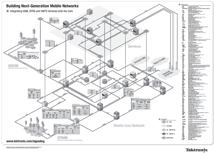
Рис. 1. Современная гетерогенная широкополосная беспроводная сеть
