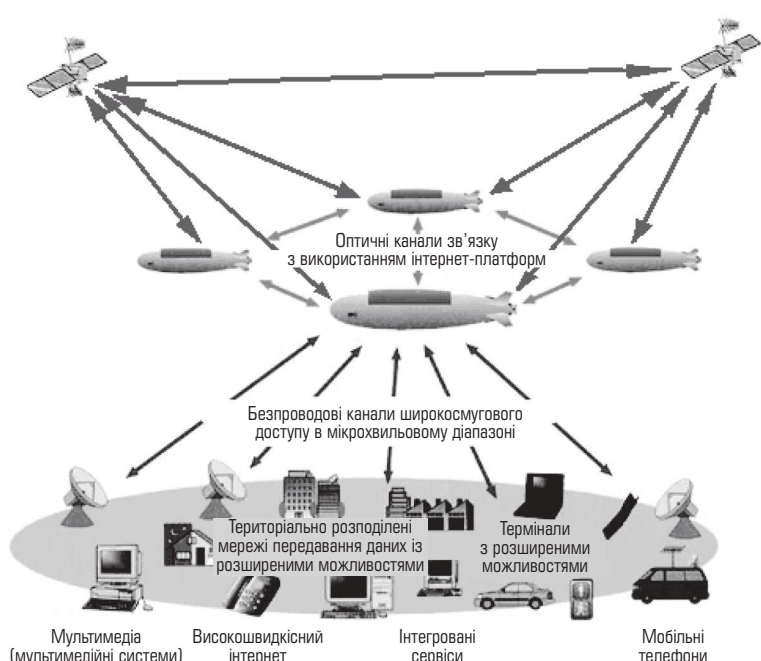
Рис. 2. Принципова схема роботи стратосферного комплексу
