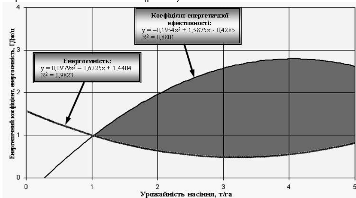
Рисунок 1. Статистична модель залежності між урожайністю насіння кукурудзи, коефіцієнтом енергетичної ефективності та енергоємністю 1 ц продукції
